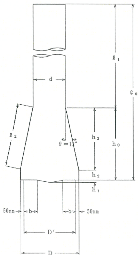
図－1 new ACE 杭の形状
